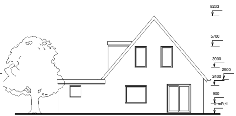
Achtergevel
