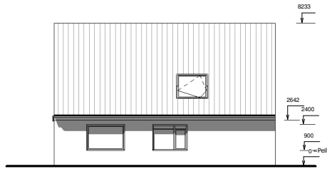
Linker zijgevel
