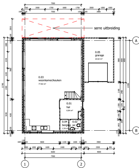
Begane Grond
