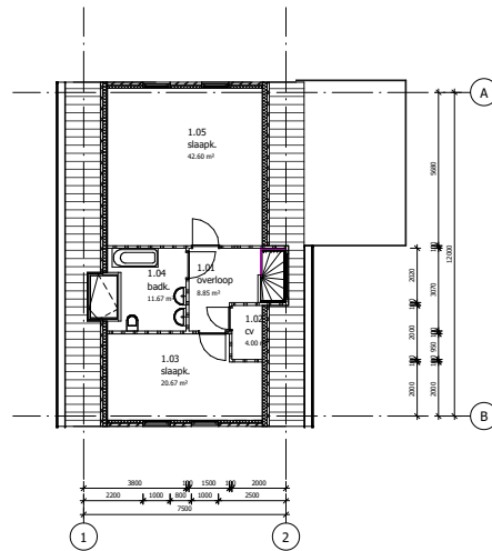
1e verdieping
