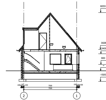
Doorsnede A-A
